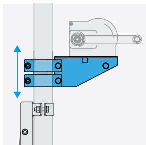
Support de treuil réglable
