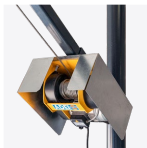
Treuil électrique avec câble acier ou Inox
